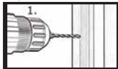
1. Pré-percer le cadre avec une mèche 5/16"
